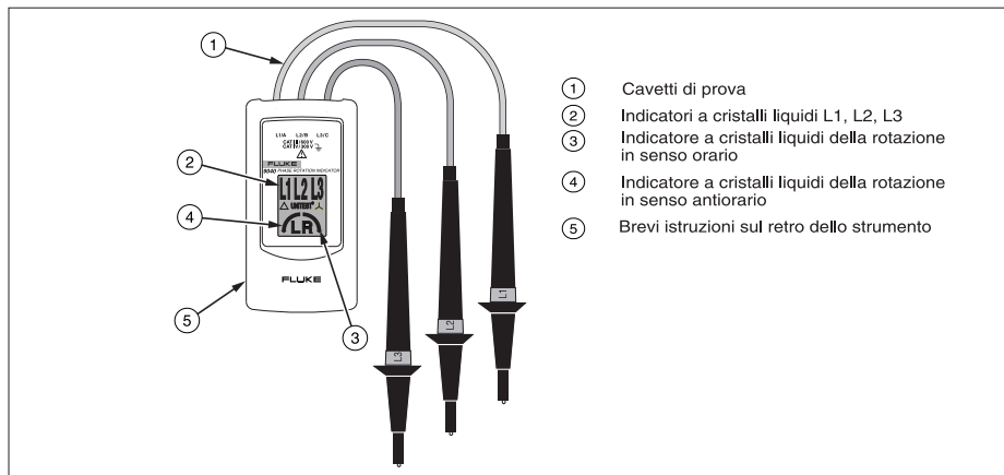
Figura 1. Il 9040 Phase Rotation Indicator
