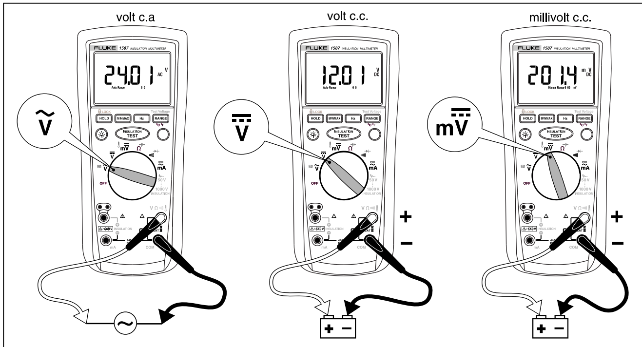
Figura 6. Misure di tensione in corrente alternata e continua
